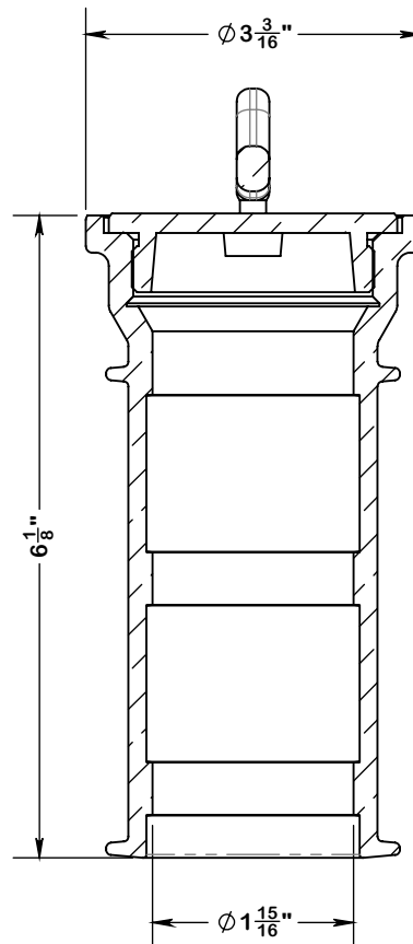
SECTION A-A
